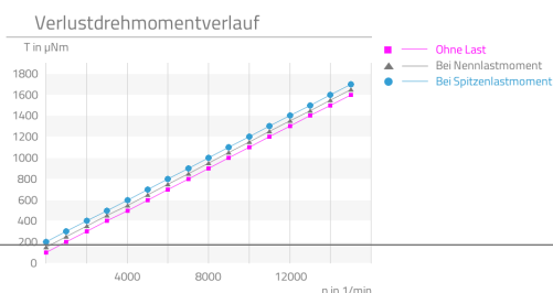
P-029 Kurve gemessen bei 5x Nennspannung mit einem Lastträgheitsmoment 6 \cdot 10E-9 kg/m 2 im \frac{1}{4} Mikroschrittbetrieb
