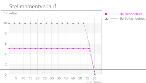
P-019 Kurve gemessen bei 5x Nennspannung mit einem Lastträgheitsmoment 6 \cdot 10E-9 kg/m 2 im \frac{1}{4} Mikroschrittbetrieb
