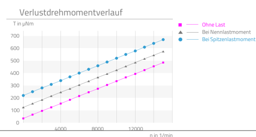
P-029 Kurve gemessen bei 5x Nennspannung mit einem Lastträgheitsmoment 6 \cdot 10E-9 \text{ kg/m}^2 im \frac{1}{4} Mikroschrittbetrieb
